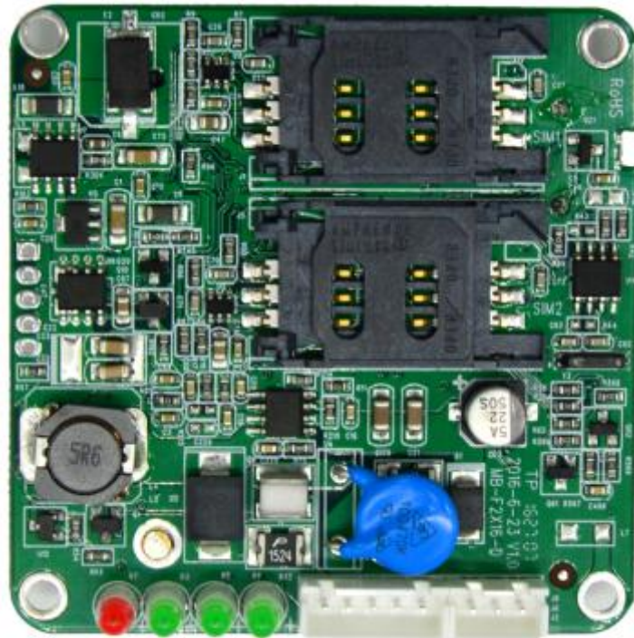
TOP 面
