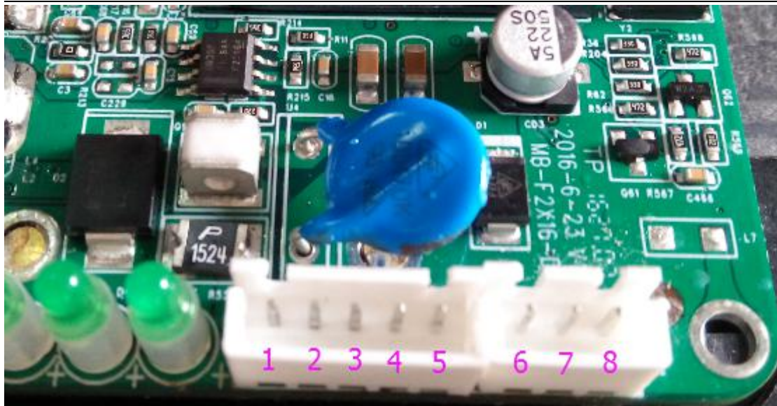
2.54mm 间距 5 针单排排母+3 针单排排母管脚定义
