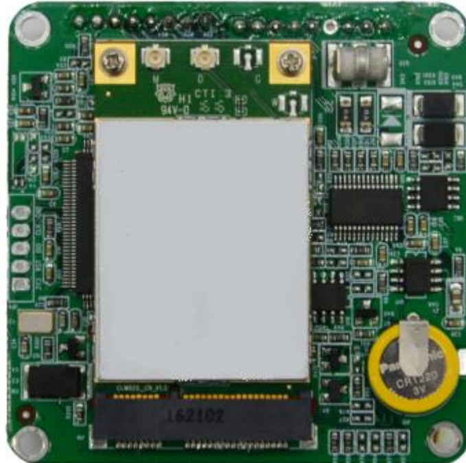
BOTTOM 面
